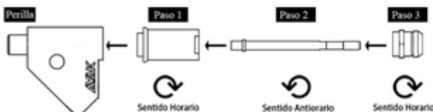
Figura 2: Instalación de accesorios para colocar tuercas/pernos remachables
