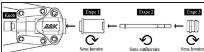
Figure 2: Installation des accessoires pour les écrous / goujons à sertir
